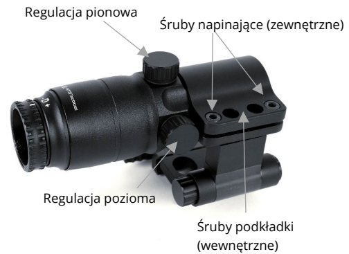
STRONA PRZEDNIA POWIĘKSZALNIKA (ta strona ma być skierowana w stronę kolimatora)
