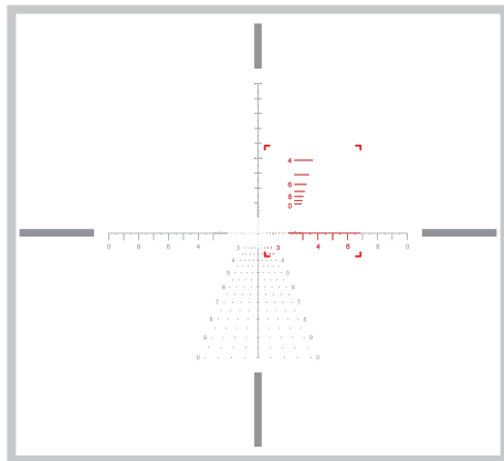
SEKCJA DRABINKI POMIARU ODLEGŁOŚCI
