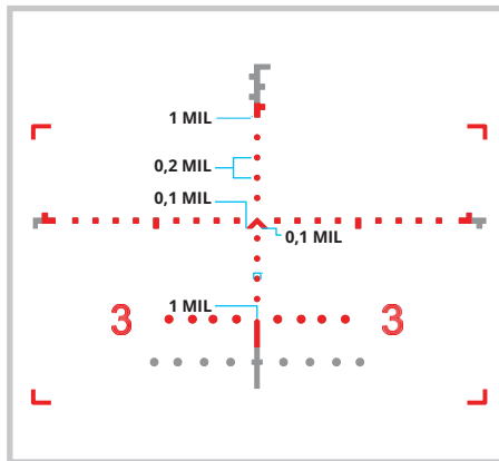
PIONOWA SEKCJA ŚRODKOWA
