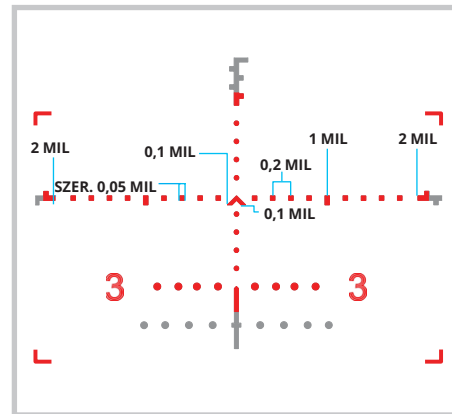
POZIOMA SEKCJA ŚRODKOWA
