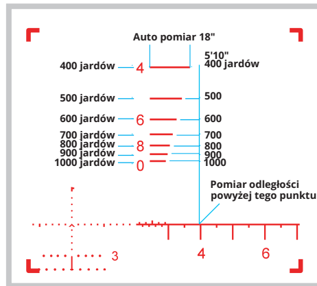
DRABINKA POMIARU ODLEGŁOŚCI
