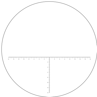
Siatka celownicza MRAD
