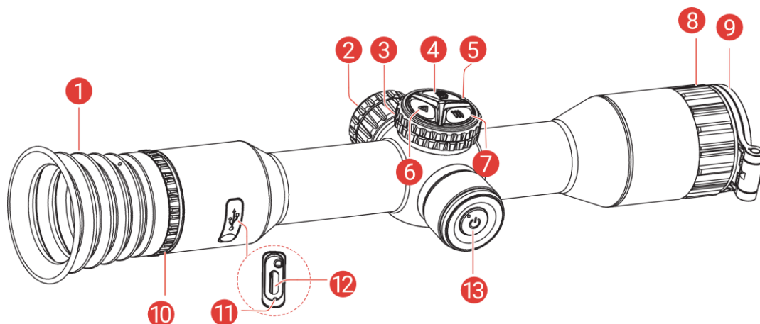
Rysunek 1-1 Wygląd modelu innego niż LRF:
