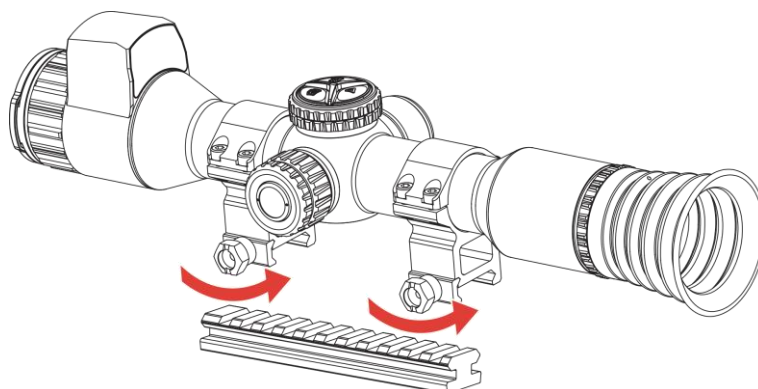
Rysunek 2-8 Odkręcanie śrub
