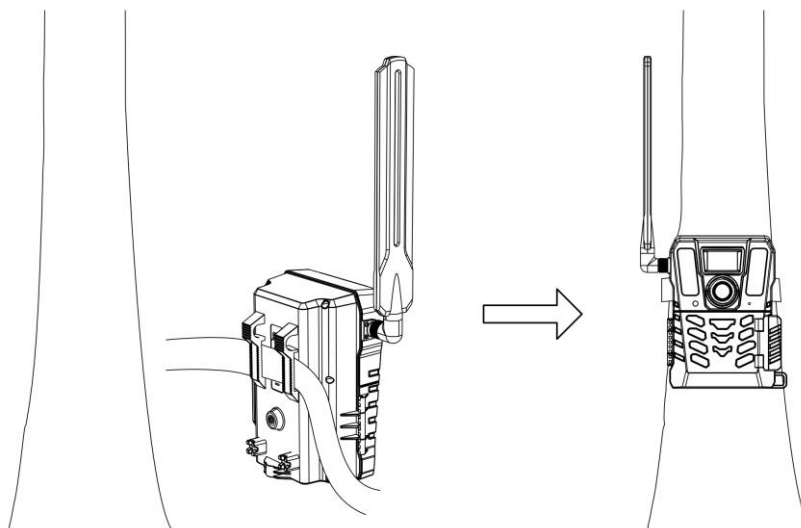
Rysunek 2-6 Instalacja urządzenia na zewnątrz
