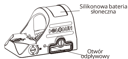
Ryc. 1 Kolimator HE507C-GR-X2
