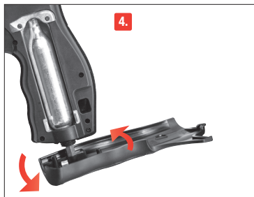
4. Вернуть прокалывающий винт для баллончика. Баллончик накаливается.
