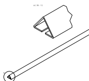
Poprzeczki do zawieszania 3 szt.
