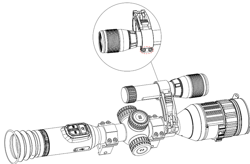
Rysunek 2-13 Mocowanie promiennika podczerwieni
