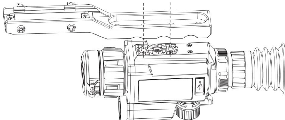
Rysunek 2-5 Ustawienie otworów instalacyjnych
