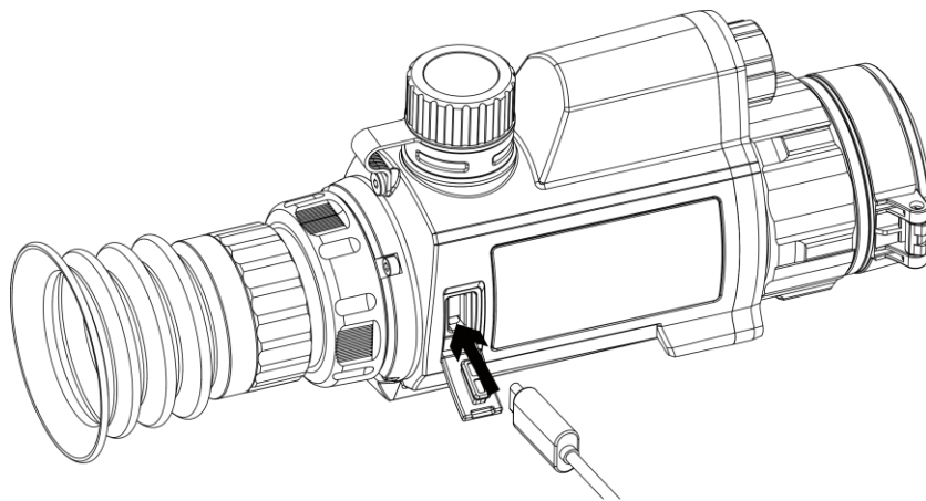
Rysunek 2-1 Podłączanie przewodów
